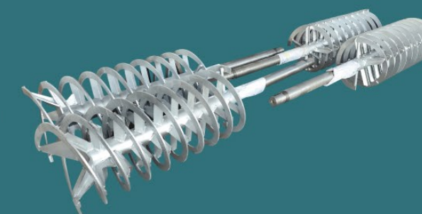
шнек ленточного податчика
